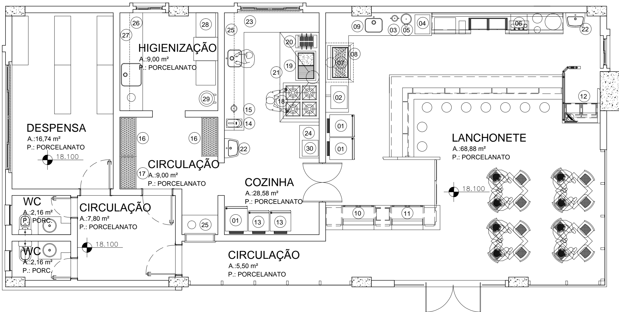
PLANTA BAIXA – LANCHONETE DO CENTRO DE ATIVIDADES
